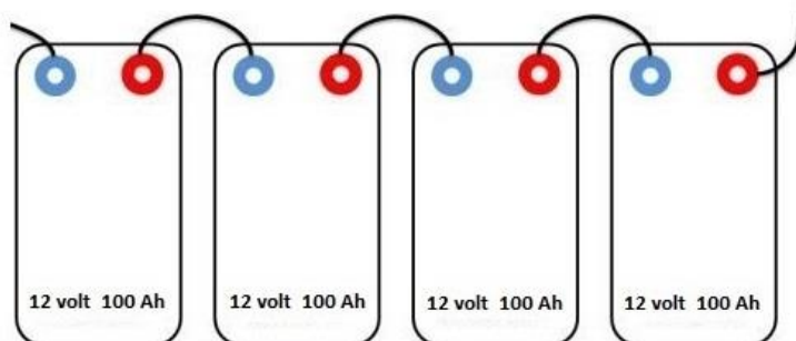
Serieschakeling 48 volt 100 Ah
