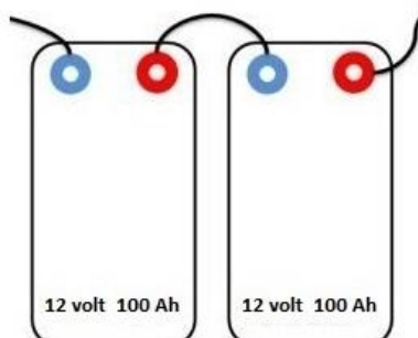
Serieschakeling 24 volt 100 Ah
