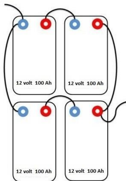
Serie- parallelschakeling 24 volt 200 Ah
