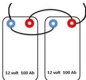
Parallelschakeling 12 volt 200 Ah
